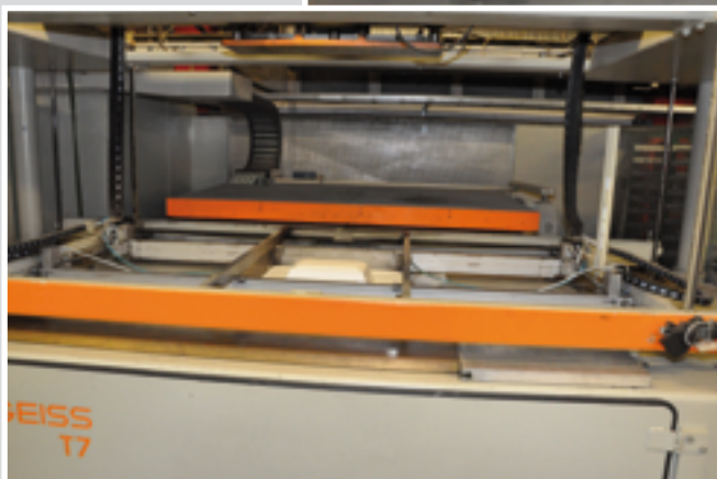
Forno per termoformatura per le cabine dell'hammam
