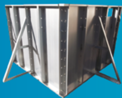
kit piscina Norin Pools in pannelli d'acciaio Magnelis
